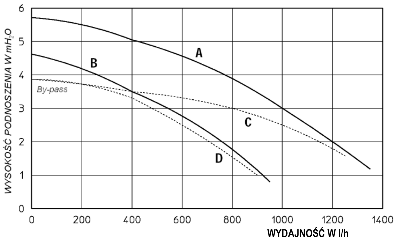
Rys. Wykres pracy pompy
