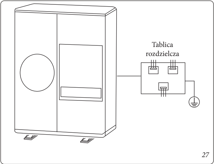
Rysunek 26: w przypadku stosowania samego zacisku uziemiającego. Rysunek 27: w przypadku korzystania z uziemienia rozdzielnic elektrycznej.
