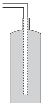
Napełnianie przy użyciu butli z dołączonym syfonem Napełnić czynnik chłodniczy z butlą w pozycji pionowej
