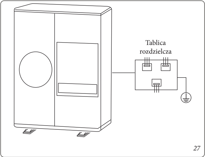
Rysunek 26: w przypadku stosowania samego zacisku uziemiającego. Rysunek 27: w przypadku korzystania z uziemienia rozdzielnicy elektrycznej.
