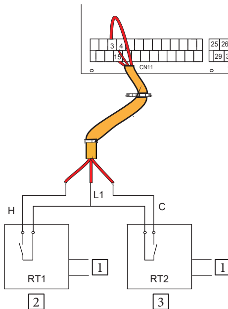
Sposób C (sterowanie dwustrefowe)
