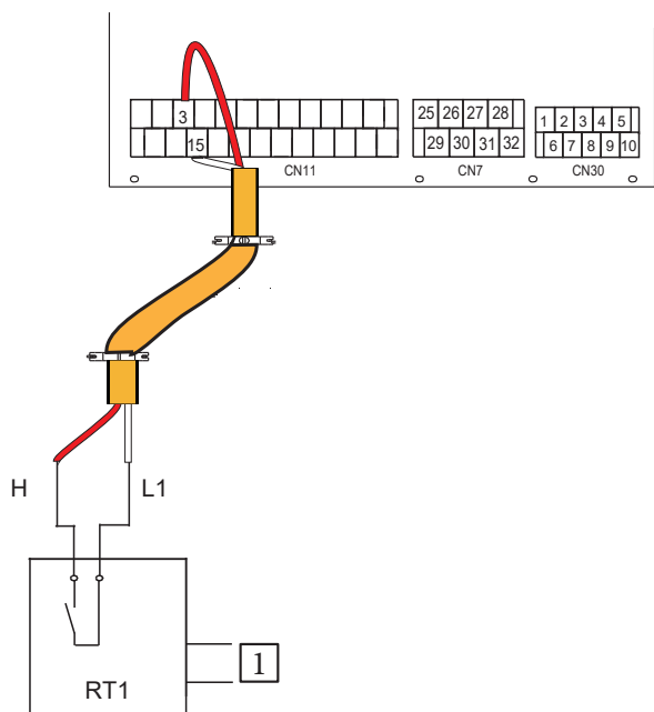
Sposób B (sterowanie jedną strefą)
