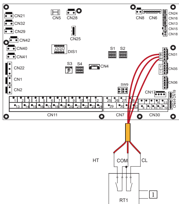
Sposób A (Sterowanie ustawionym trybem)
