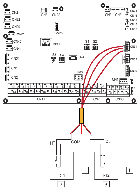
Sposób C (sterowanie dwustrefowe)
