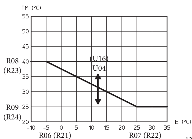
Temperatura zasilania w strefie 2 (3) mieszanej w fazie chłodzenia i obecności sondy zewnętrznej
