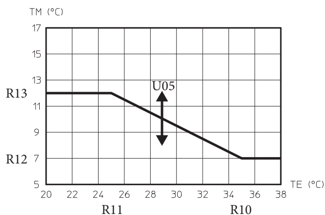
Temperatura zasilania w fazie c.o. bez sondy zewnętrznej
