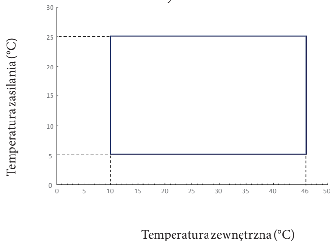
Ograniczenia działania pompy ciepła w trybie chłodzenia
