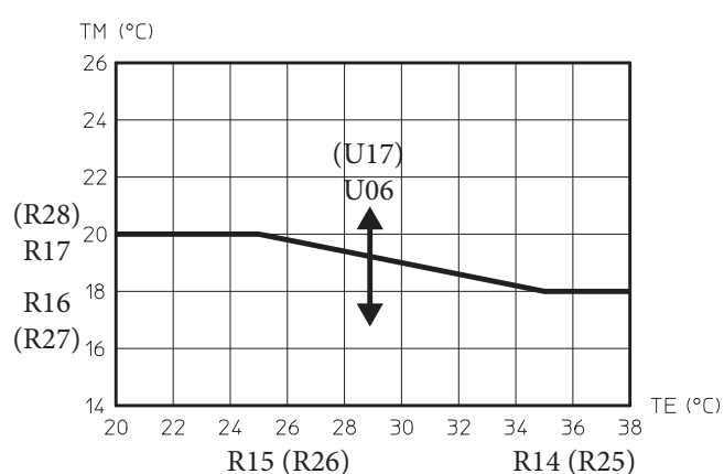
Temperatura zasilania w strefie 2 (3) mieszanej w fazie chłodzenia i obecności sondy zewnętrznej
