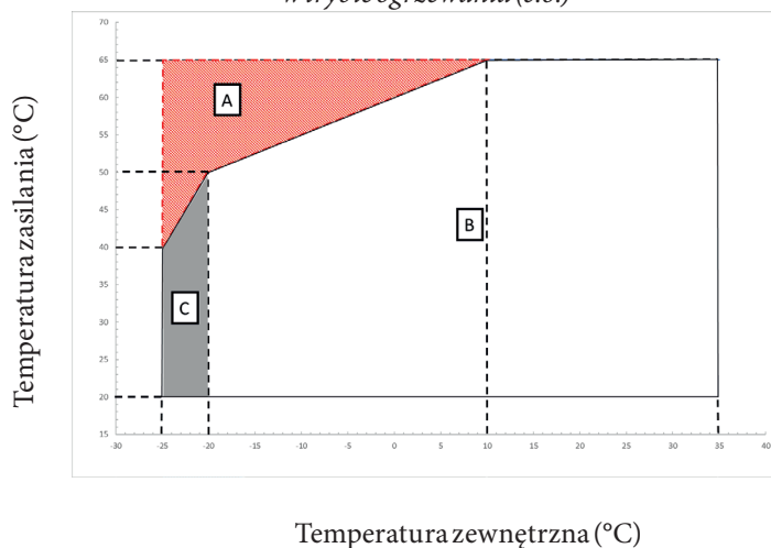
Ograniczenia działania pompy ciepła w trybie ogrzewania (c.o.)
