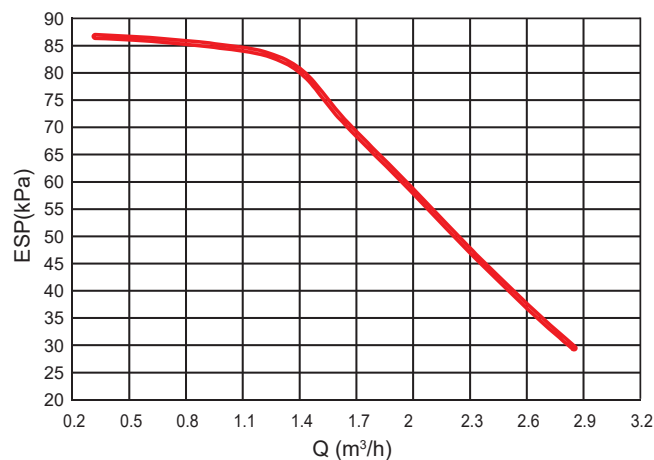
Dostępne zewnętrzne ciśnienie statyczne VS Natężenie przepływu 4-6 kW
