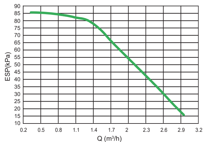
Dostępne zewnętrzne ciśnienie statyczne VS Natężenie przepływu 8-10 kW
