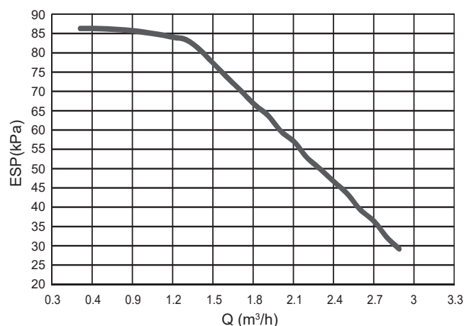
Dostępne zewnętrzne ciśnienie statyczne VS Natężenie przepływu 12-14 kW
