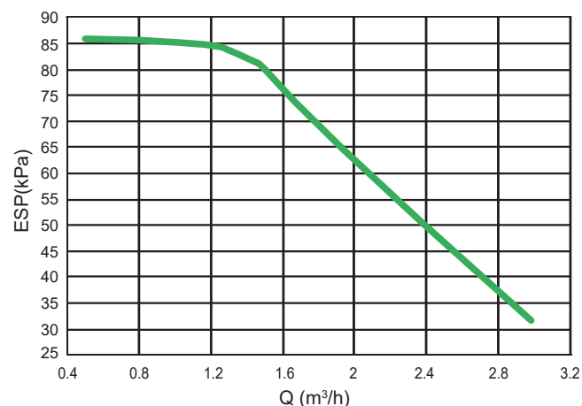
Dostępne zewnętrzne ciśnienie statyczne VS Natężenie przepływu 16 kW
